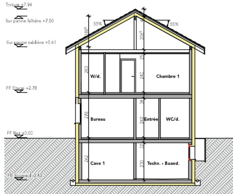
Coupe A-A
